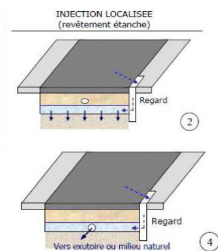
Exemples de structure réservoir - Source 2LM
